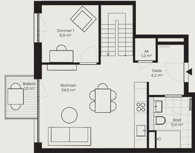
4.OG
